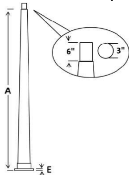
Detalle del Niple
