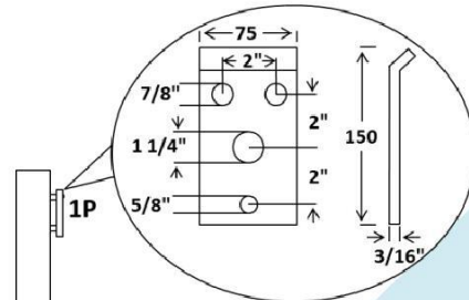
Detalle de la Percha
