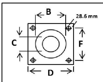
Detalle de la Placa Base
